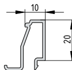
ЭК-4061
