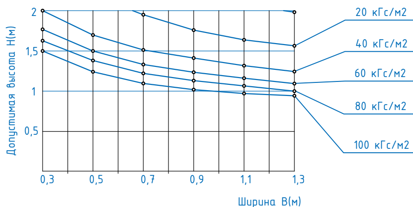
График предельного соотношения высоты и ширины створки ЭК-6990 в зависимости от ветрового района
