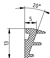
ТПУ-004ММ ( M=0.055\text{кг/м} )
