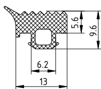
ТПУ-002ММ ( M=0.083\text{кг/м} )
