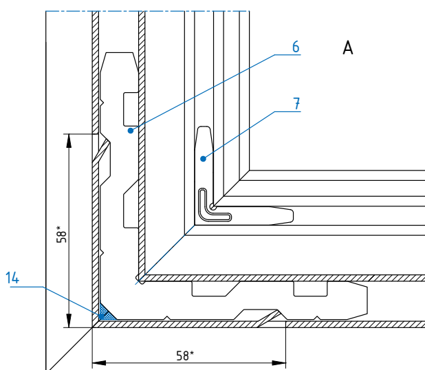
Сборка угла на закладной ЭК-4050
