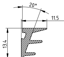
ТПУ-1042
