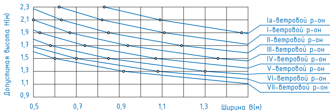
График предельного соотношения высоты и ширины створки ЭК-6990 в зависимости от ветрового района
