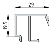
ТП-5093
