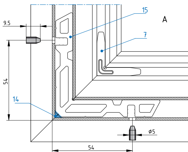
Сборка угла на закладной ЭК-4050
