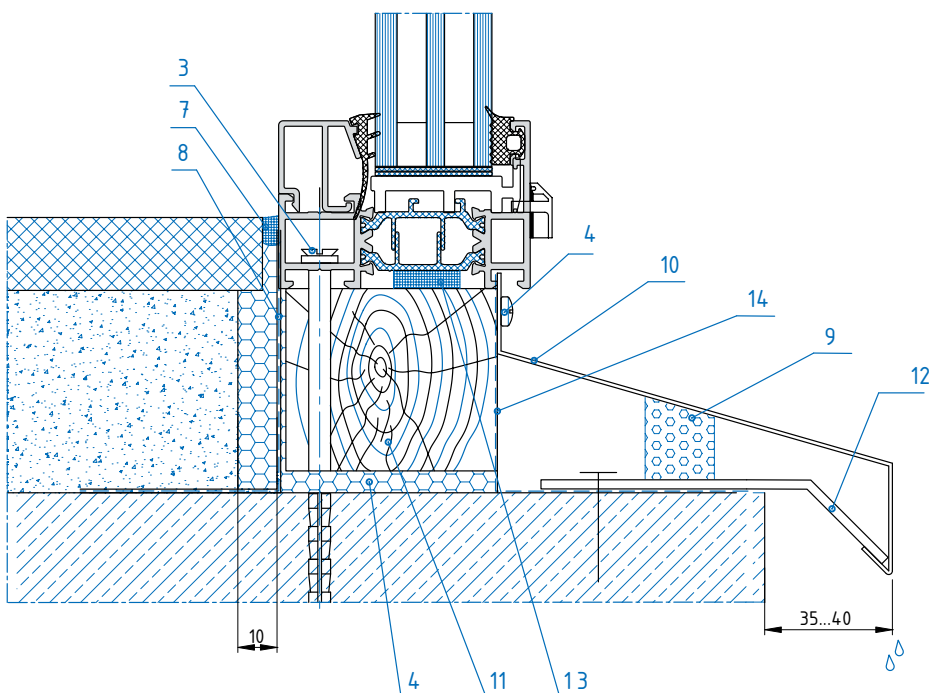
Б-Б Узел нижнего примыкания
