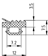
ТПУ-6001 ( M=0.066 \text{ кг/м} )
