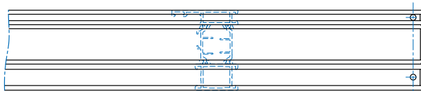
Обработка нижнего ригеля рамы ЭК-6911 ПХ.03.071.001.004
