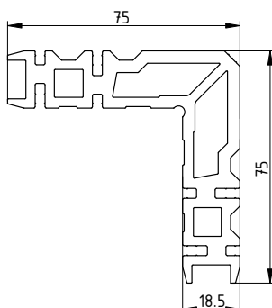
ТП-45.08.03 L=8,5мм
