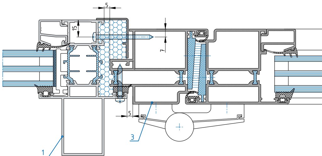
В-В (открытие наружу)
