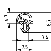
ТПУ-006-01ММ ( M=0.031\text{кг/м} )
