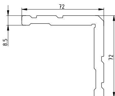
ТПТ-66205
