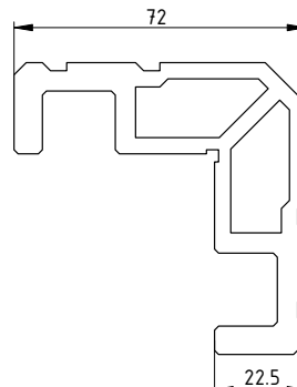
ТП-5034 L=8,5мм L=17,5мм
