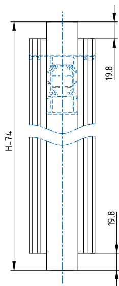
Обработка импосты рамы ЭК-6920 ПХ.03.071.001.005
