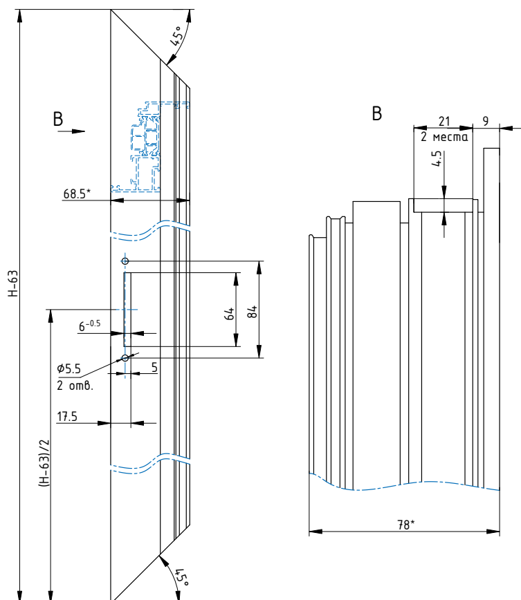
Обработка стойки створки ЭК-6930 ПХ.03.071.002.001
