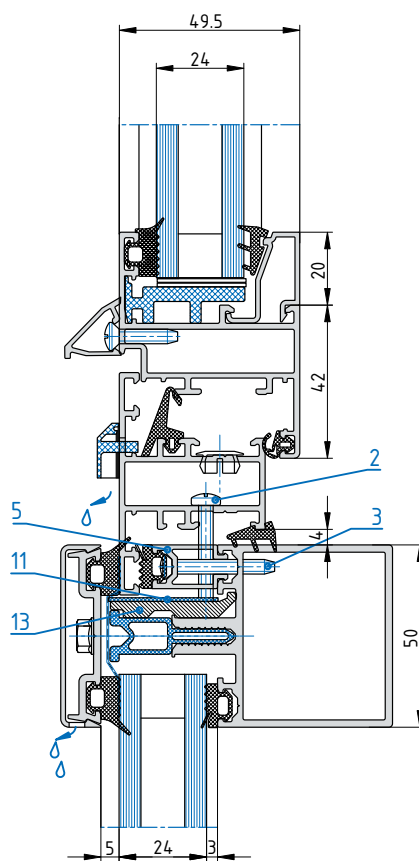
Б-Б СПО-24мм
