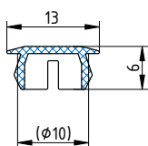
ТПУ-021
