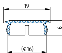
ПХ.02.015.000.003 Пробка
