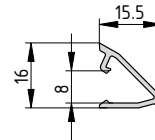
ЭК-4080
