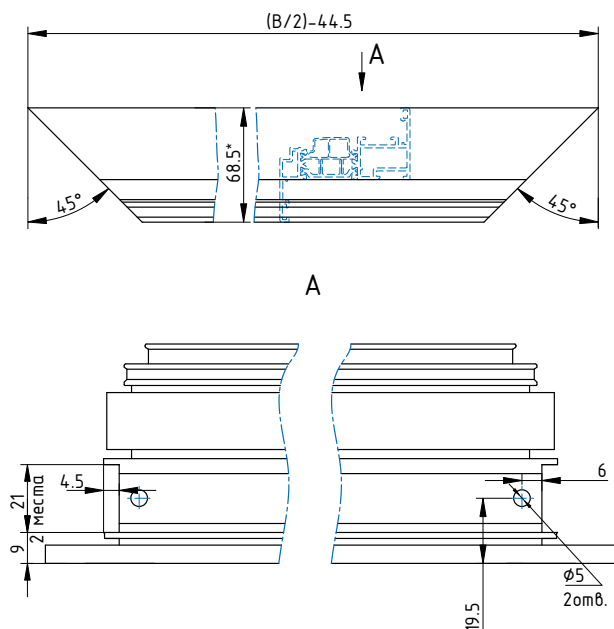
Обработка верхнего ригеля створки ЭК-6930 ПХ.03.071.002.003
