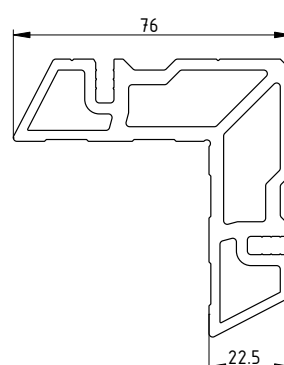
ТП-45.08.04 L=8,5мм L=17,5мм
