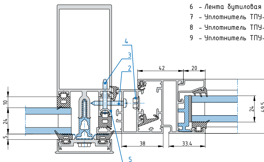
A-A СПО-24мм
