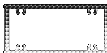
ТП-5013-02 L=33мм
