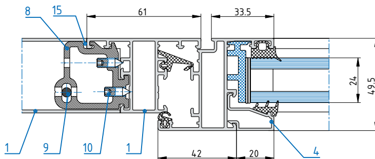
А-А СПО-24мм
