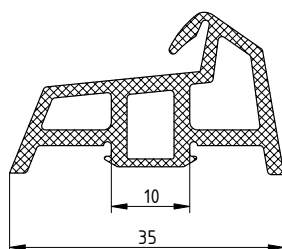
ТПУ-6901 ( M=0.258\text{кг/м} )
