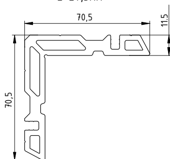
ТП-45.08.02 L=8,5мм L=18,5мм L=27,5мм
