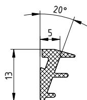
ТПУ-004ММ ( M=0.055 \text{ кг/м} )
