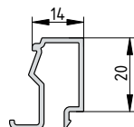
ЭК-4060
