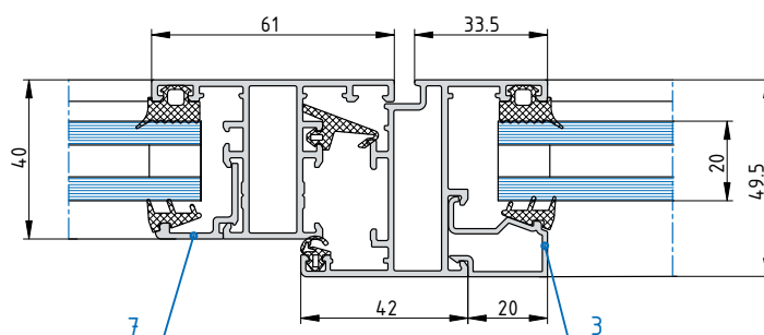
Б-Б СПО-20мм
