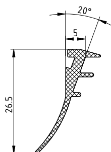
ТПУ-004-01 ( M=0.075\text{кг/м} )
