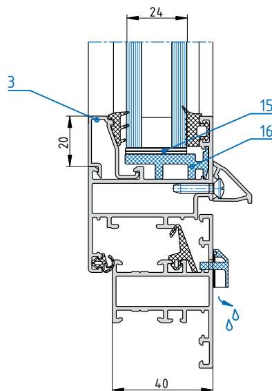
Б-Б СПО-24мм
