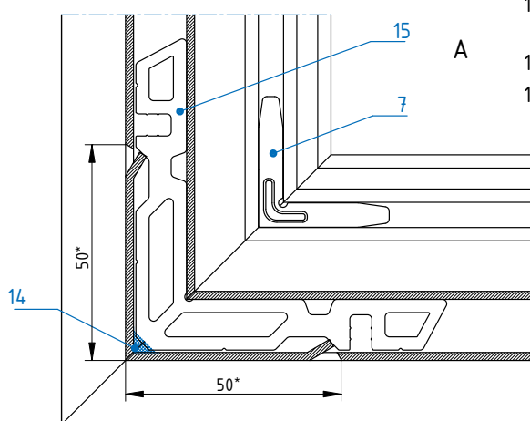
"Нагельное" соединение угла на закладной ТП-45.08.02
