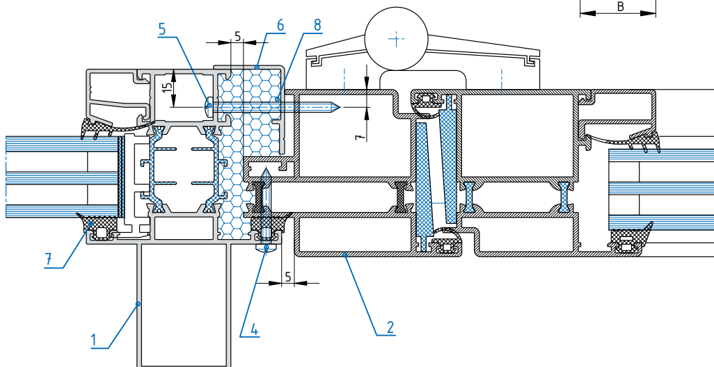
В-В (открытие наружу)
