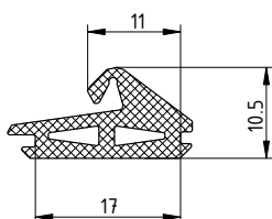
ТПУ-8901 ( M=0.113 \text{ кг/м} )
