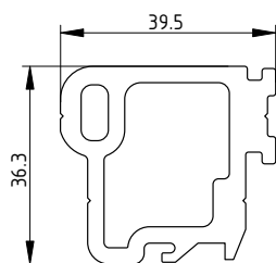
ЭК-40103 L=11,5мм
