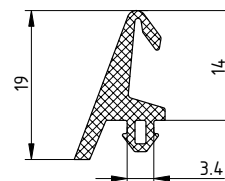
ТПУ-4005 ( M=0.09\text{кг/м} )
