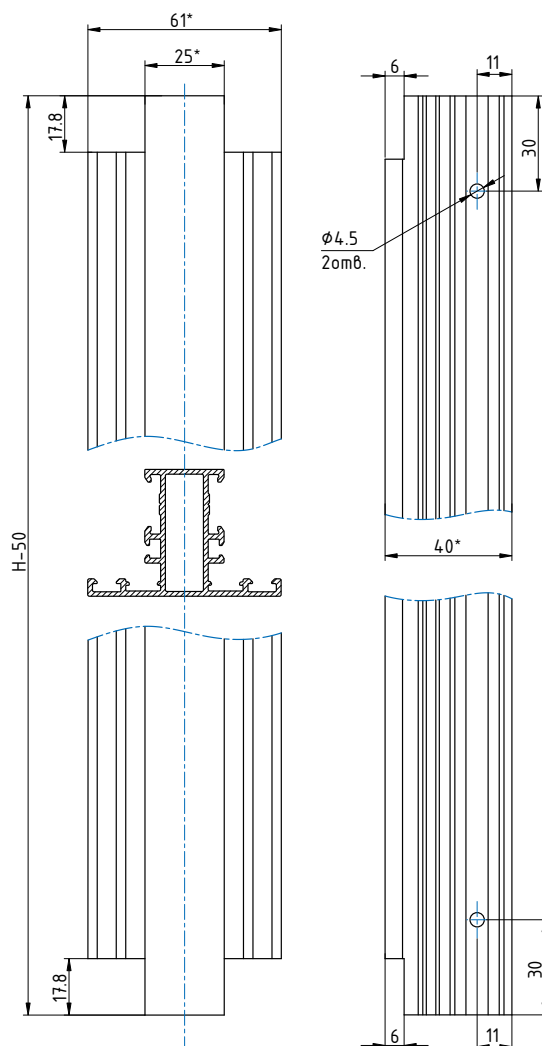
Обработка средней стойки ЭК-4020
