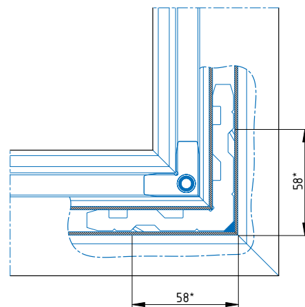
Обжимка угла створки
